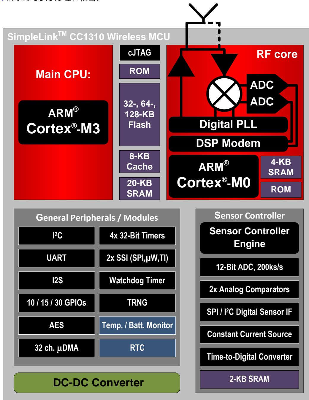
图 1-1. CC1310 框图
