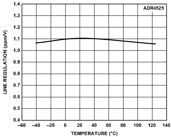
图22. ADR4525线性调整率与温度的关系
