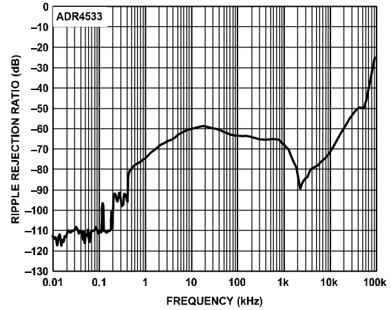
图53. ADR4533纹波抑制比与频率的关系
