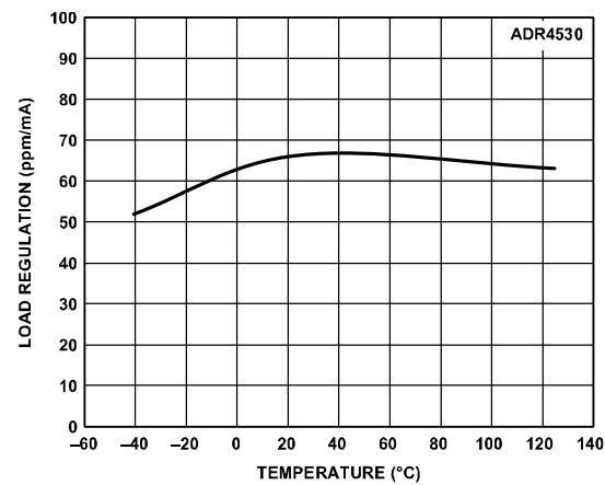
图35. ADR4530负载调整率与温度的关系 (吸电流)
