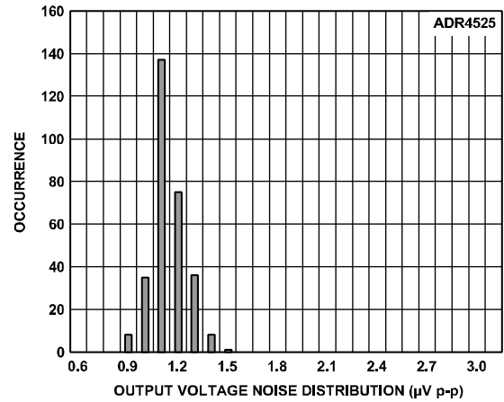
图24. ADR4525输出电压噪声 (最大幅度从0.1 Hz到10 Hz)
