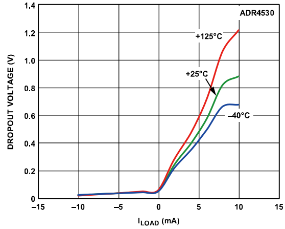
图33. ADR4530压差与负载电流的关系
