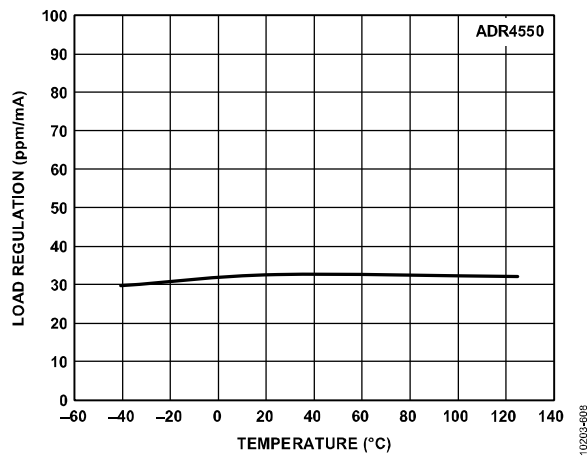
图74. ADR4550负载调整率与温度的关系 (吸电流)
