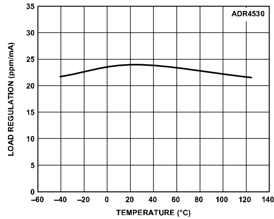
图34. ADR4530负载调整率与温度的关系 (源电流)
