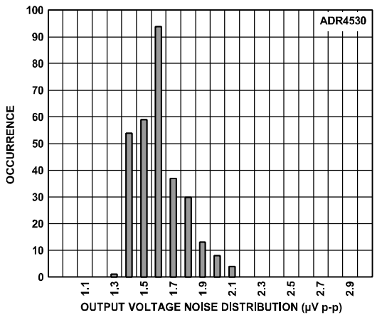
图38. ADR4530输出电压噪声 (最大幅度从0.1 Hz到10 Hz)
