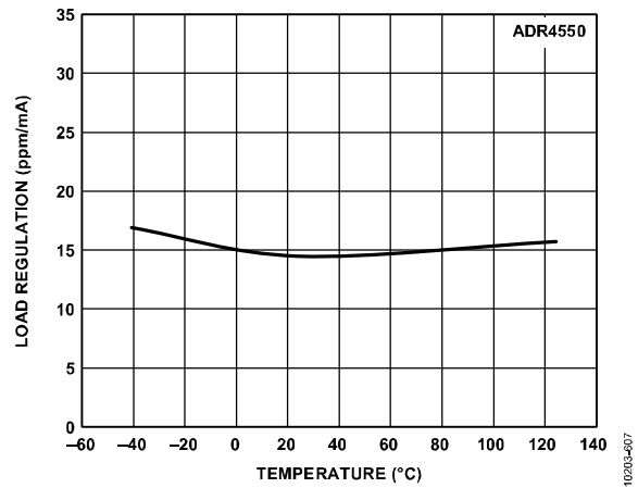
图73. ADR4550负载调整率与温度的关系 (源电流)
