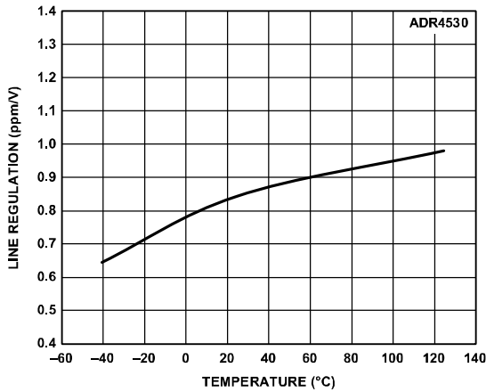
图36. ADR4530线性调整率与温度的关系
