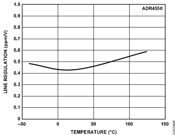
图75. ADR4550线性调整率与温度的关系
