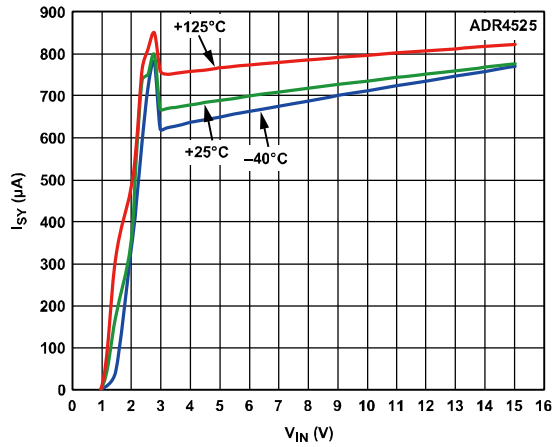
图23. ADR4525电源电流与电源电压的关系
