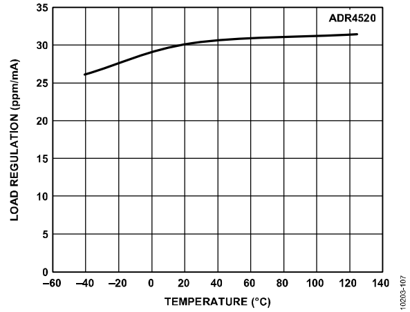
图6. ADR4520 负载调整率与温度的关系 (源电流)
