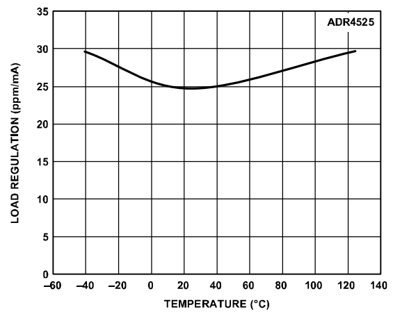
图20. ADR4525负载调整率与温度的关系 (源电流)
