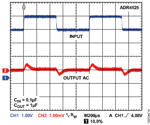
图27. ADR4525线路瞬态响应
