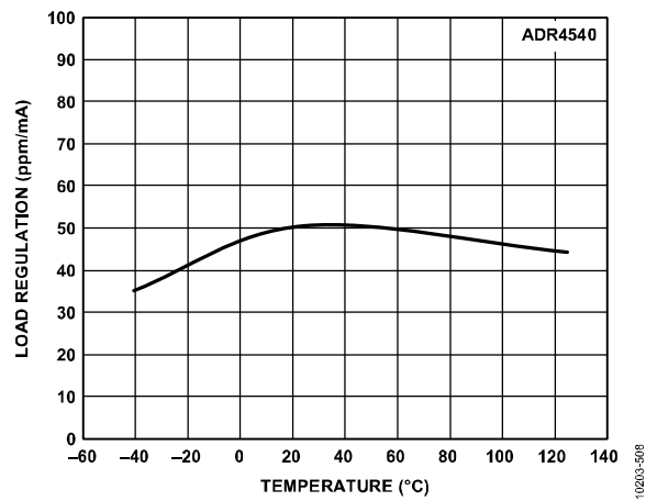
图61. ADR4540负载调整率与温度的关系 (吸电流)
