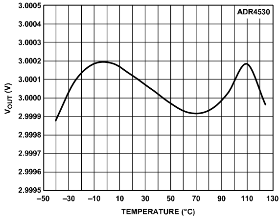
图30. ADR4530 B级输出电压与温度的关系
