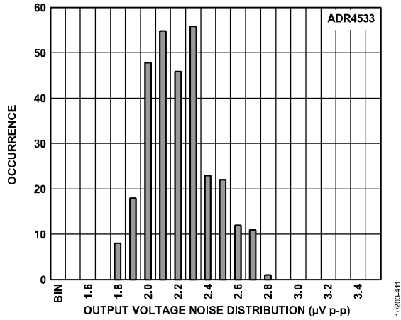
图51. ADR4533输出电压噪声 (最大幅度从0.1 Hz到10 Hz)
