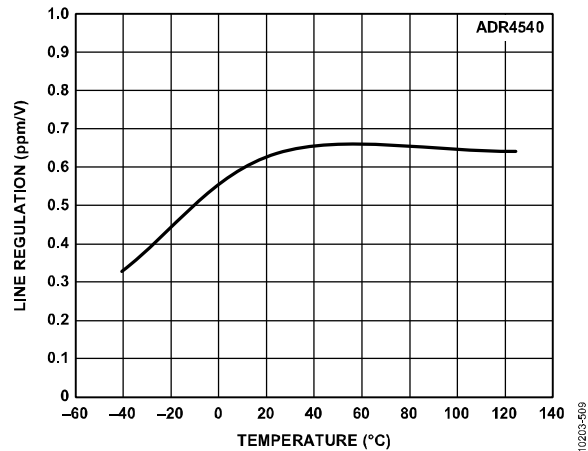
图62. ADR4540电源电压调整率与温度的关系
