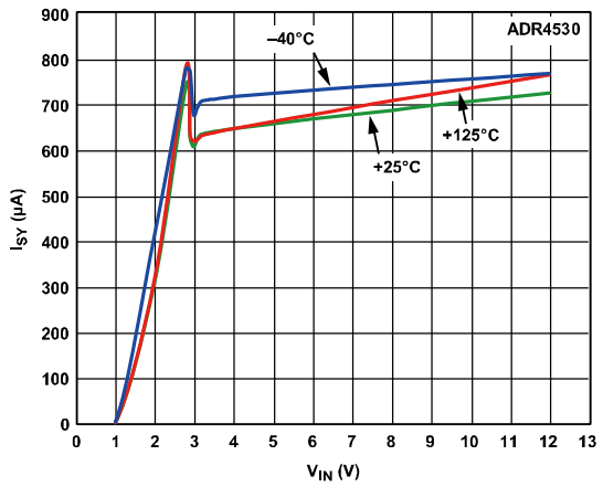
图37. ADR4530电源电流与电源电压的关系
