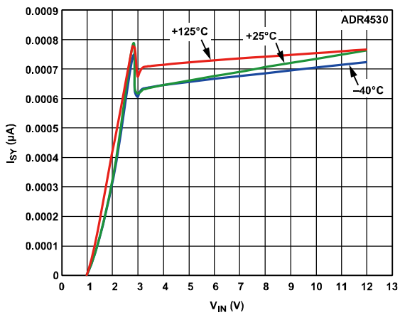
图32. ADR4530电源电流与电源电压的关系
