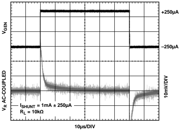
图9. ADR5041瞬态响应
