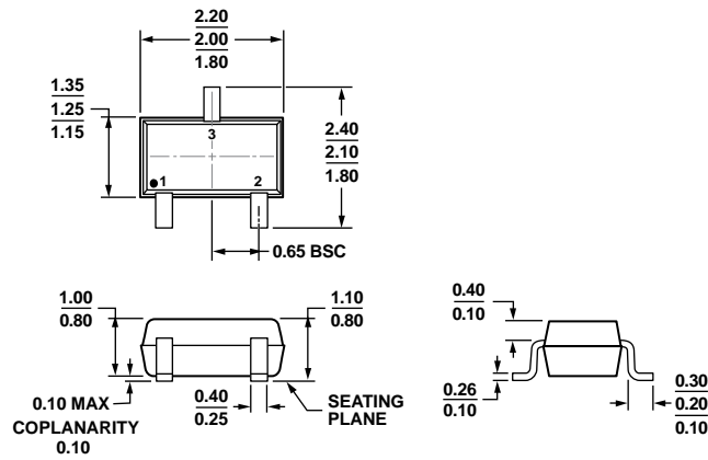
图24. 3引脚超薄紧缩小型晶体管封装[SC70] (KS-3)
