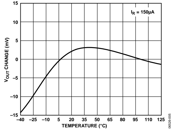
图5. ADR5045 V_{OUT} 变化与温度的关系
