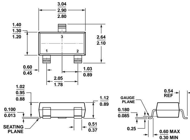
图25. 3引脚小型晶体管封装[SOT-23-3] (RT-3)
