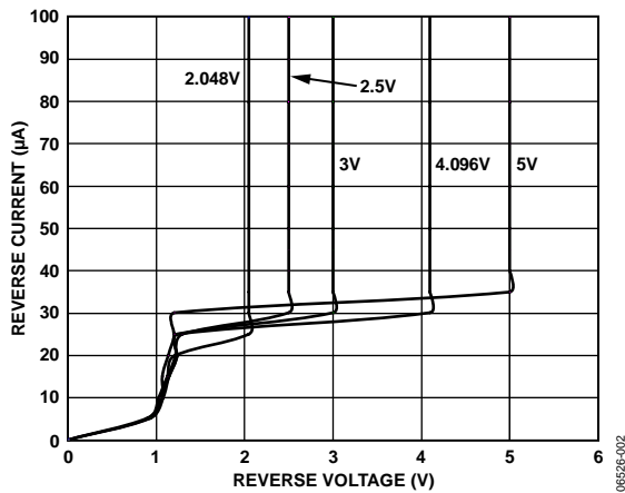
图16. ADR504x反向特性和最小工作电流
