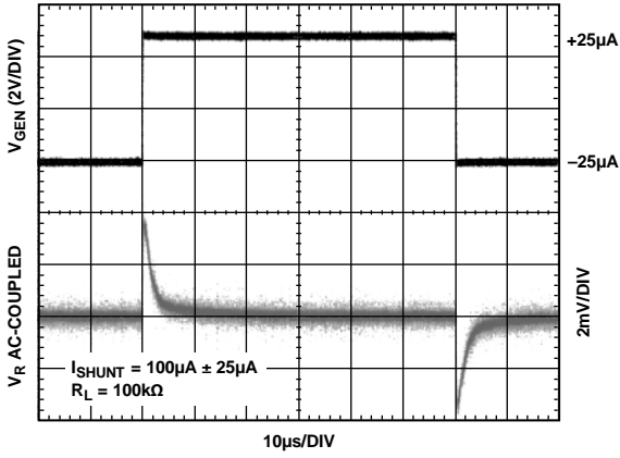
图8. ADR5041负载瞬态响应
