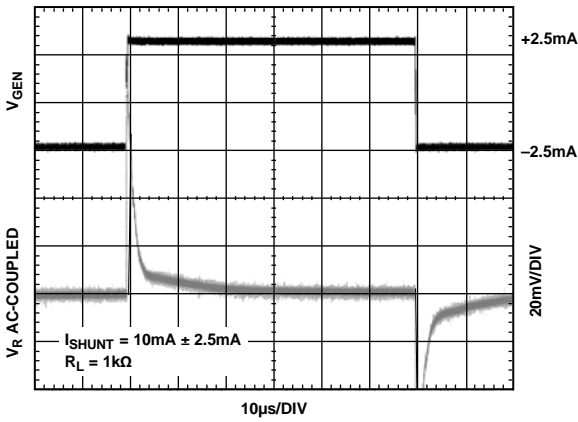
图10. ADR5041瞬态响应
