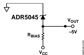
图20. 负精密基准电压配置
