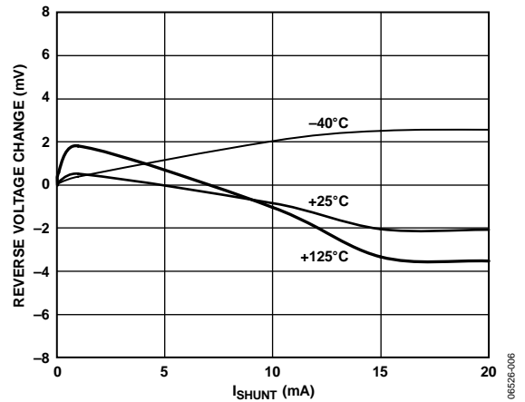
图6. ADR5045反向电压变化与 I_{SHUNT} 的关系
