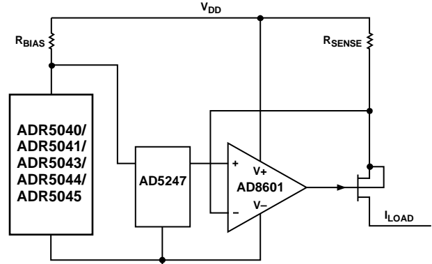
图23. 可编程电流源
